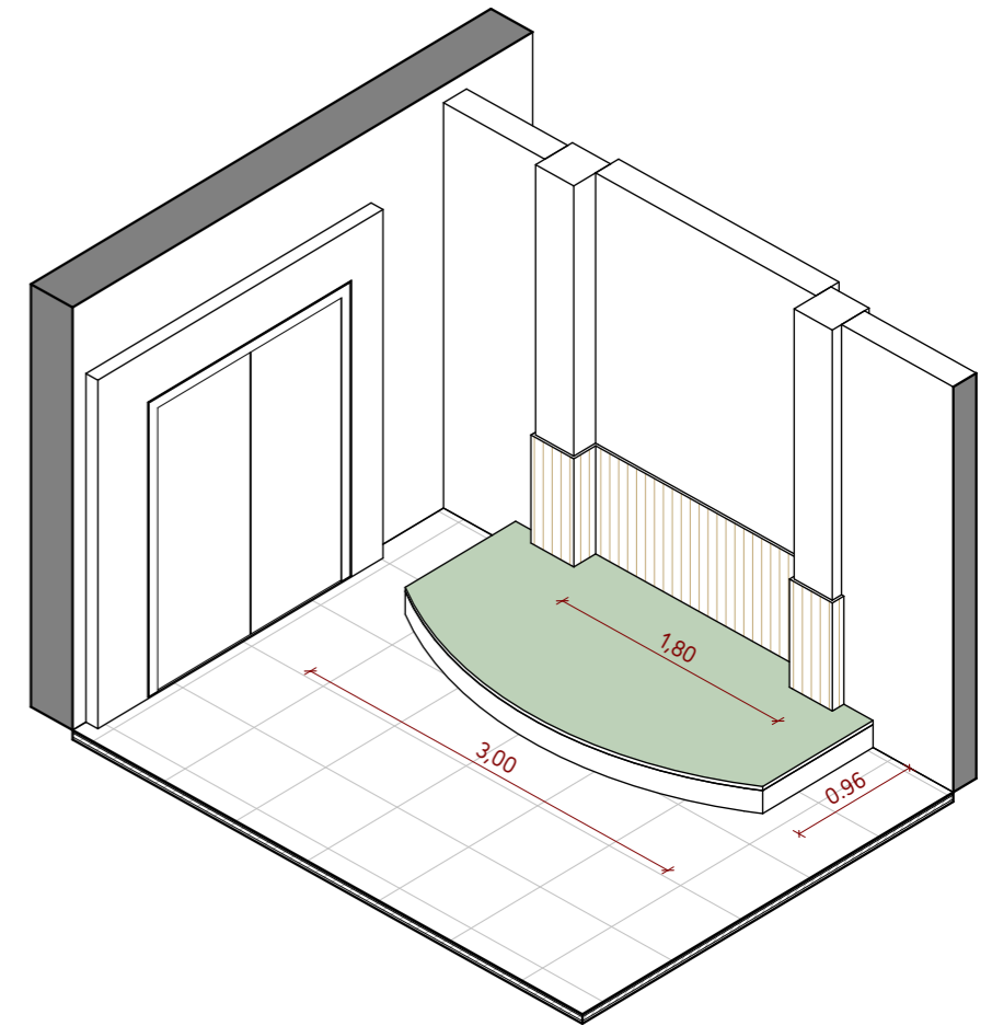
DETALLE. Axonometría escenario.
